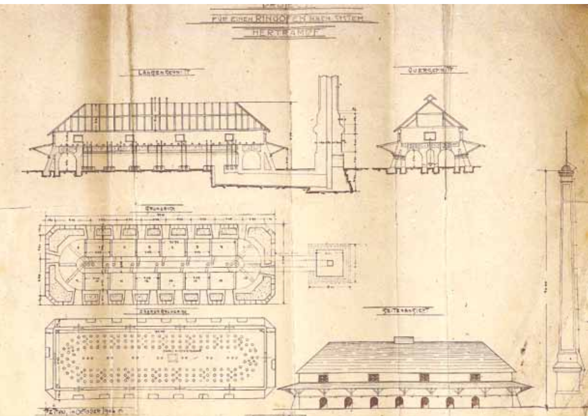
Slika 1: Načrt za opekarno po sistemu Hertrampf, ki je bila predvidena za lokacijo v Janežovcih (ZAP, Drava načrti, predal št. 1, ovoj 15)
