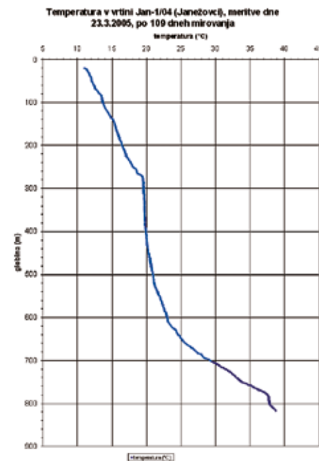
Slika 3: Termokarotaža vrtine Jan-1/04 dne 23. marca 2005
