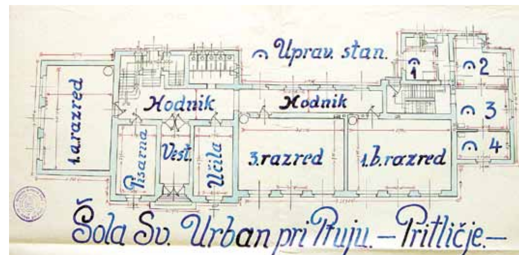
Slika 2: Tloris prvega nadstropja šole
