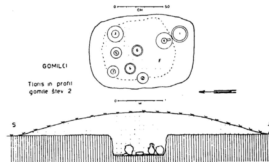
Slika 3: Gomilci, profil in tloris gomile 2
