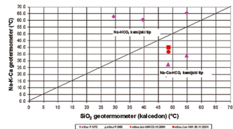
Slika 2: Relativna primerjava izračunanih geotermometrov
